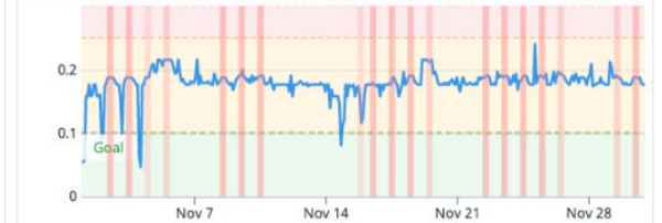
CLS - Cumulative Layout Shift (P75)
